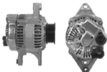
14857 100211-2102 12V/80A
