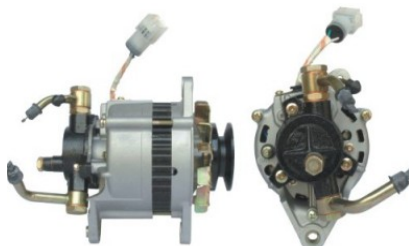
12097 12V/70A 204-329 LR170-418
