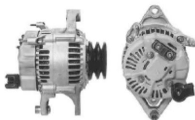
13305 121000-3310 12V/90A
