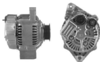
13331 100211-8300 12V/80A
