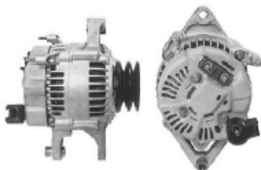
13306 121000-3390 12V/90A
