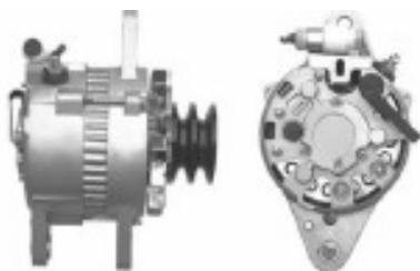
8-97361-871-0 12V/90A LR190-763
