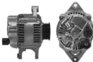
13924 121000-4360 12V/125A
