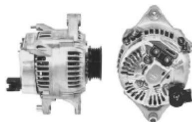
13301 121000-4040 12V/120A
