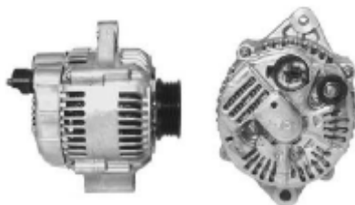
12066 100211-6030 12V/120A
