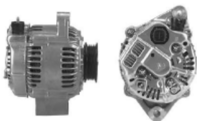
13424 100211-8530 12V/80A
