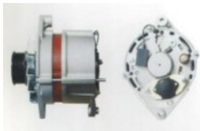
12376 CA1393IR 24V/120A 0120689517 0120689522
