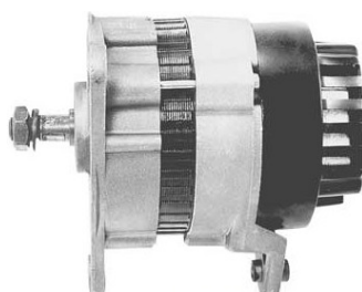
20182 24V/35A LRA02447
