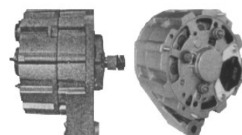
CA568IR 24V/30A 0120489316
