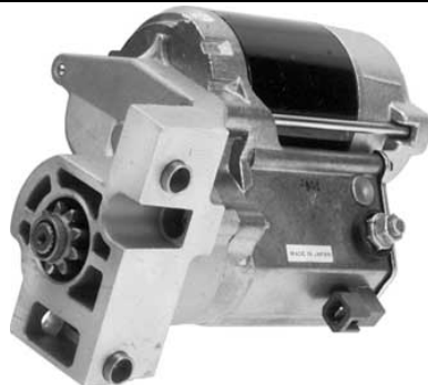
2-1561-ND 17546 12V/1.4KW/9T/CW 228000-0810
