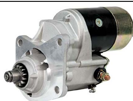
QD6236A 18507 228000-7300 12V/2.5KW/13T
