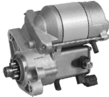
17671/17707 2-1837-ND 12V/1.4KW/9T/CW 228000-5300
