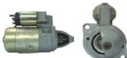
LESTER: 17770 F-005-M00-004 12V/1.4KW/9T
