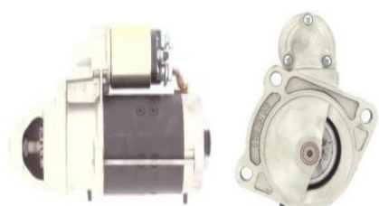
0001-231-034/023 24V/4.0KW/11T
